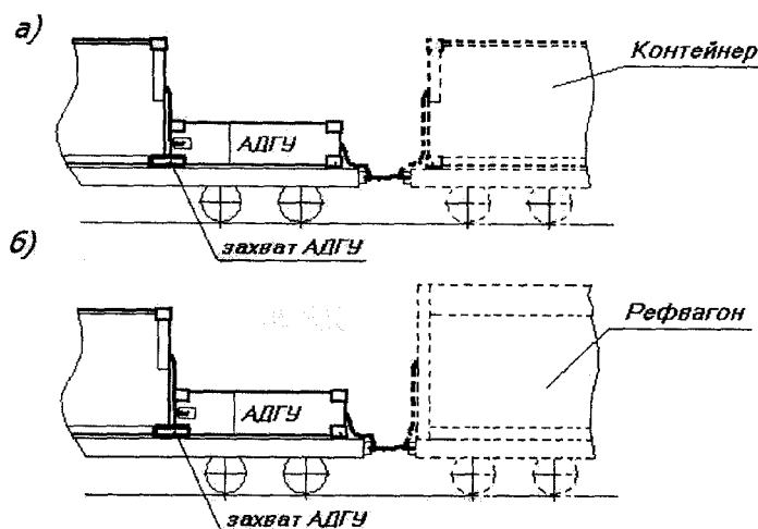
Рисунок 17 «АДГУ» - «Прогрессор-1» или РКВ-15
