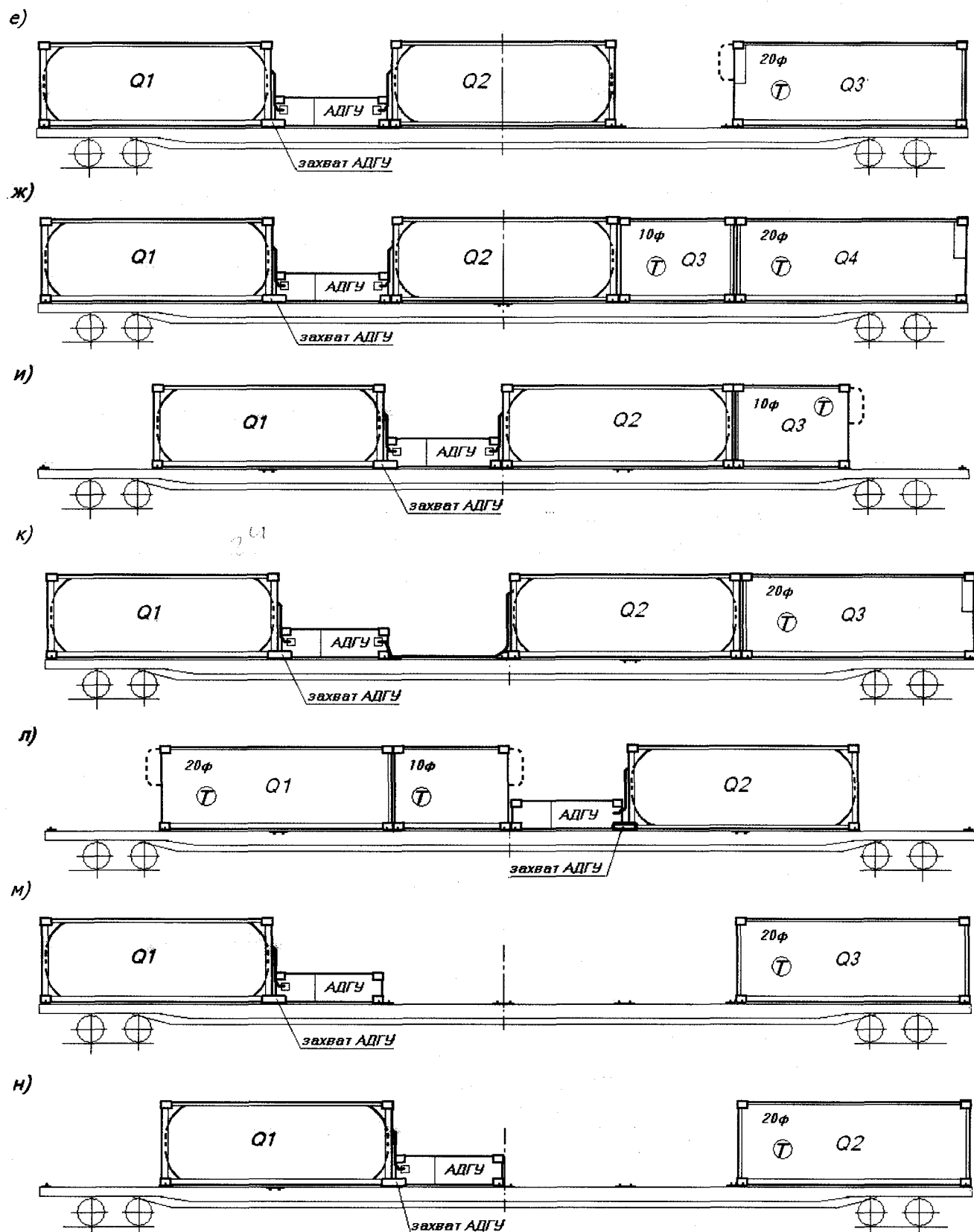
Рисунок 19 (продолжение) «АДГУ» - «Прогрессор-1» или РКВ-15
