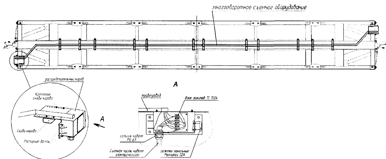
Рисунок 3 – Многооборотное съемное оборудование по проекту 4728-10.00.00.000
