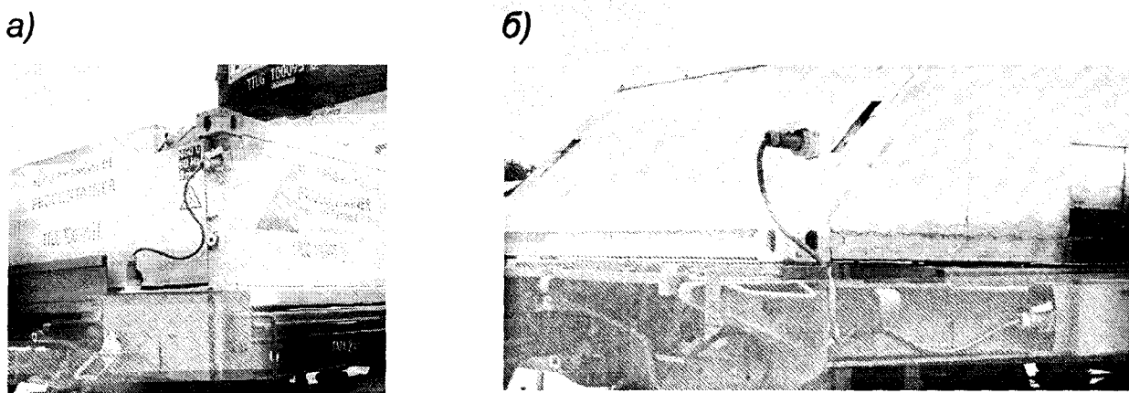
Рисунок 17-1 - Подключение АДГУ к сети электроснабжения платформы а – подключение АДГУ «Прогрессор-1»; б – подключение АДГУ РКВ-15
